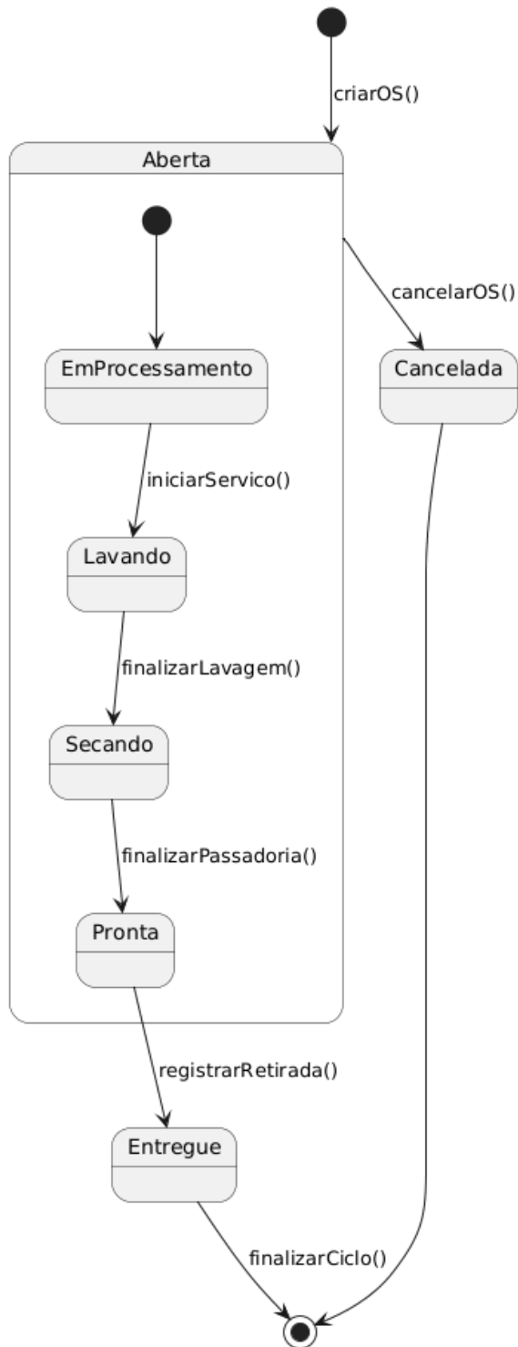
Diagrama de Estados - Ordem de Serviço (OS)
