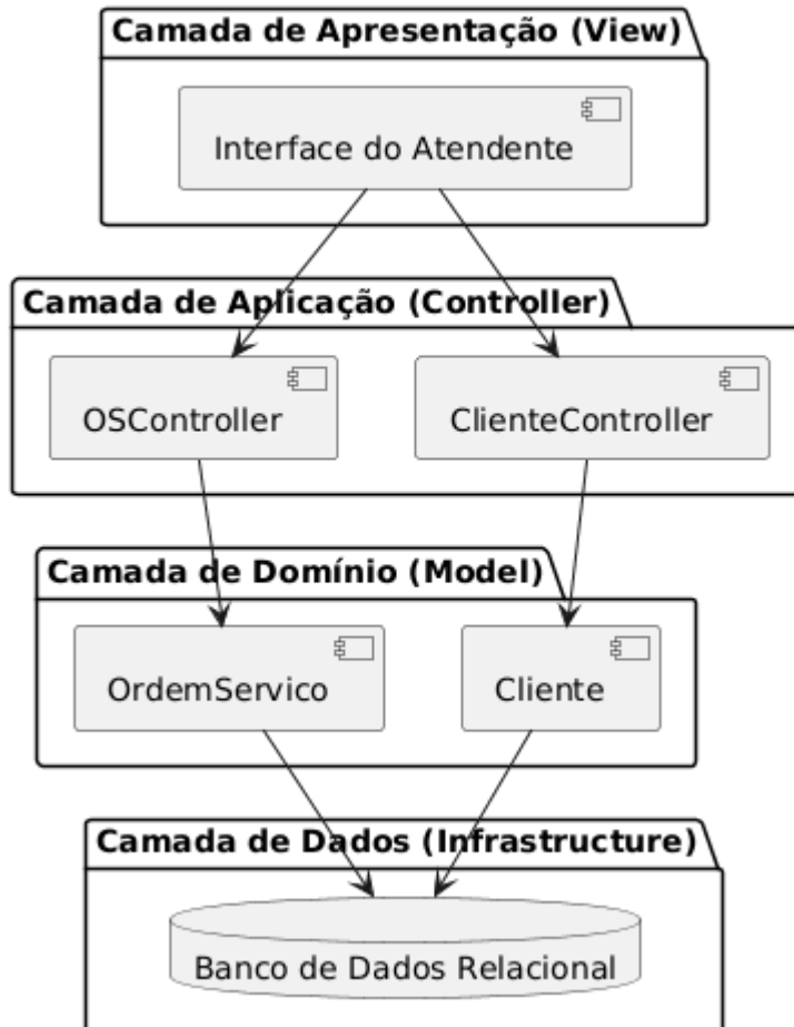
Diagrama de Arquitetura - Lavanderia Express
